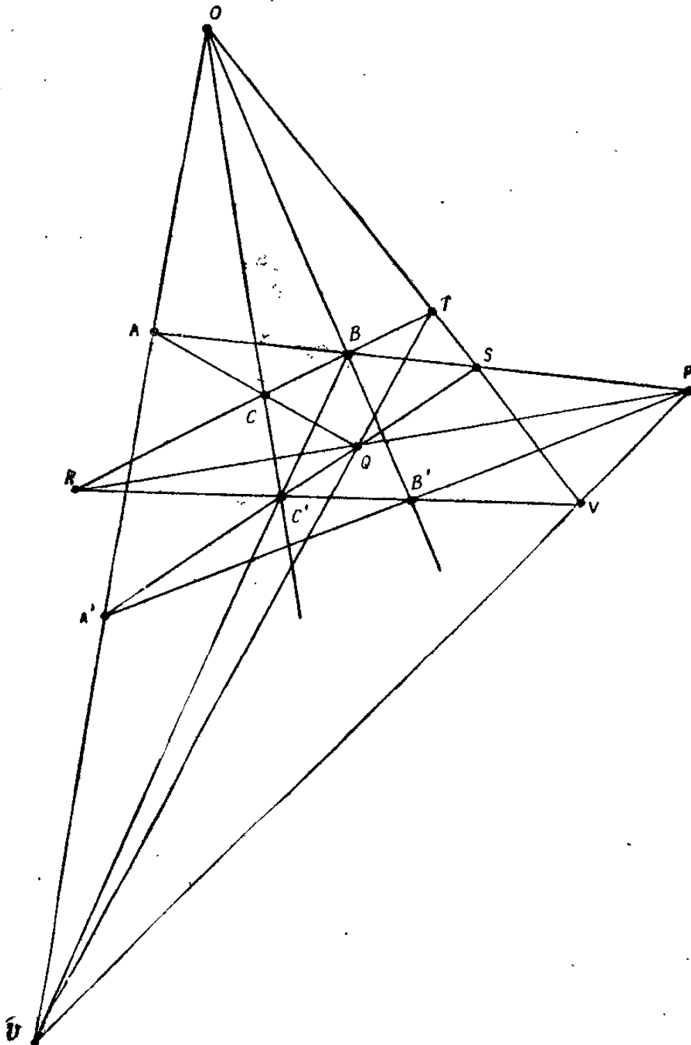
Рис. 33. Аксиома Паппа \Rightarrow Аксиома Дезарга.
